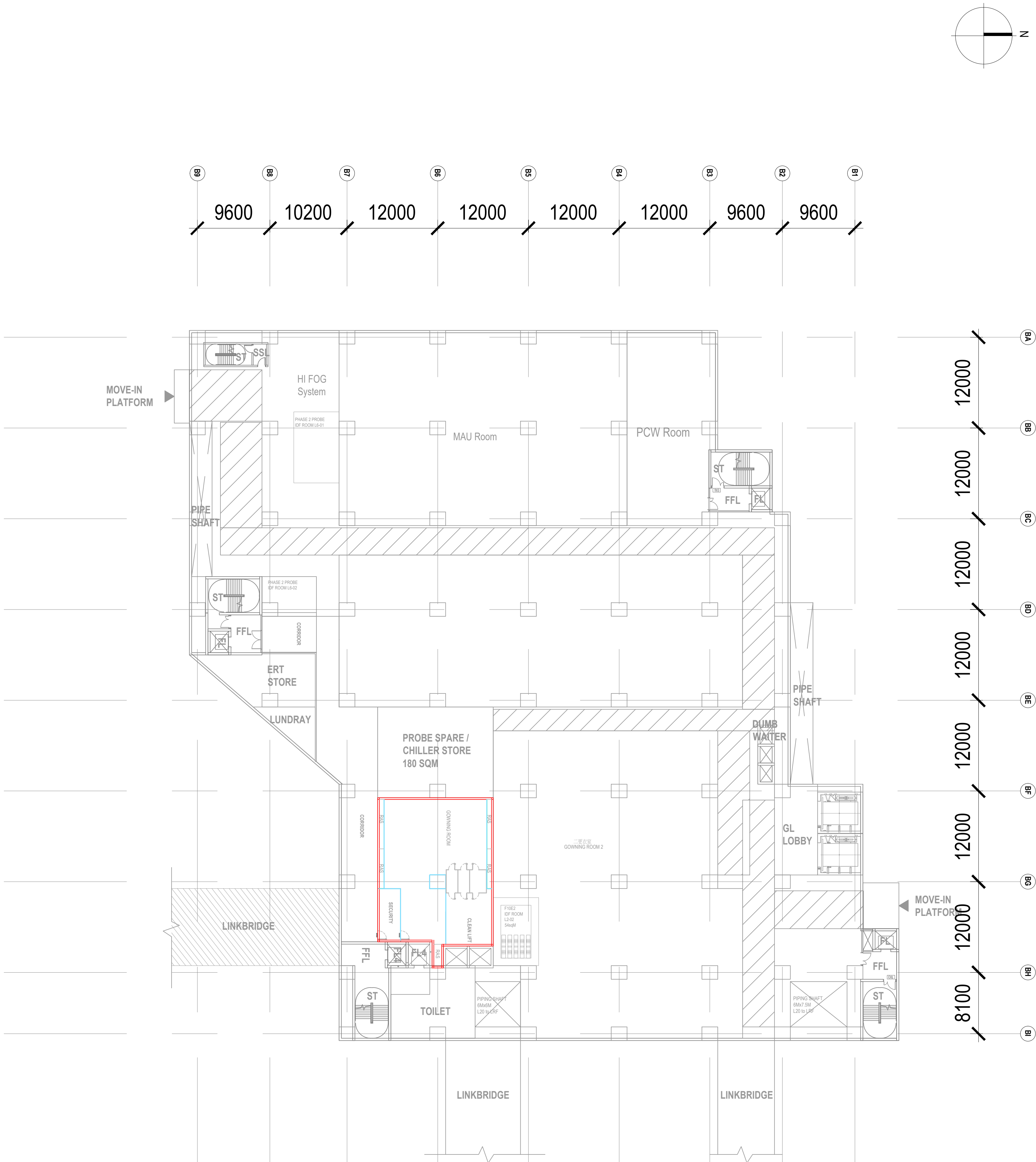
F10E2 L20 PARTITION LAYOUT SCALE 1:300
